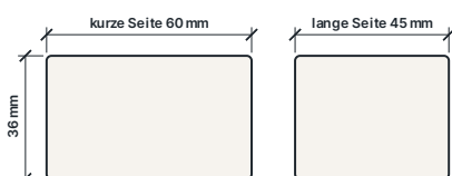
Querschnitt des Profils – schematisch.
